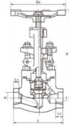
主要外形尺寸及连接尺寸mm)
