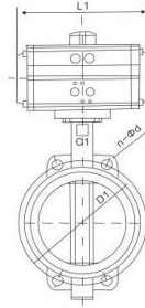
尺寸size(mm)
